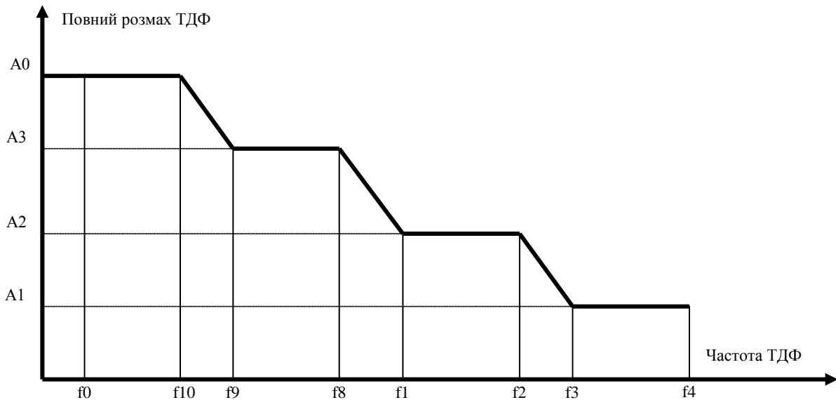
Рис. 2. Допустимі тремтіння і дрейф фази на входах інформаційних інтерфейсів
